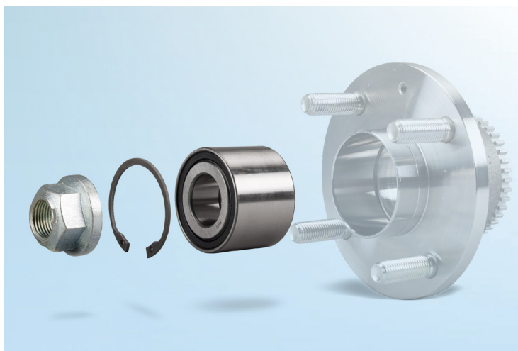
תמונה מס' 1: קיט מיסב הגלגל של FAG 713 6448 00 כפתרון לצורך תיקון – אין להחליף טבור הגלגל מושלם.
