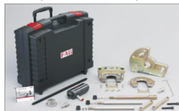
Рис. 2: Специальный инструмент 400 6199 10 обязателен при монтаже подшипника.
