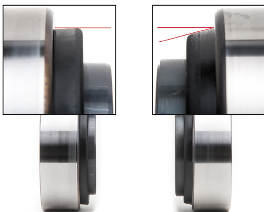
Fig. 1: Forma constructivă a capacului de protecție împotriva prafului a fost modificată
