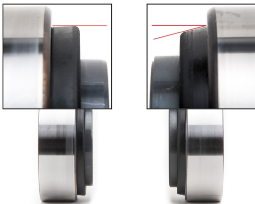
Εικόνα 1: Ο σχεδιασμός του προστατευτικού καλύμματος σκόνης άλλαξε
