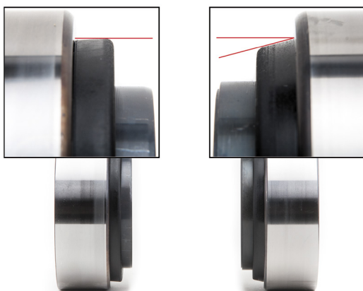
1. ábra: Módosították a porvédő sapka kialakítását
