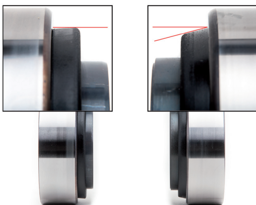
Figura 1: il design del parapolvere è stato modificato
