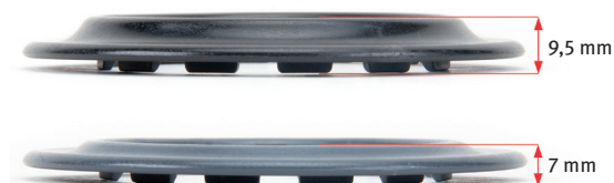
Fig. 1: Los dos anillos de protección se diferencian únicamente en la altura
