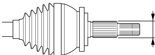
Figura 1: Pentru identificarea rulmentului de roată corect, măsurați diametrul exterior al arborelui canelat al articulației homeocinetice
