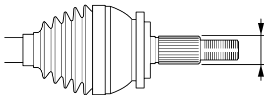
Bild 1: Zur Identifizierung des korrekten Radlagers ist der Außendurchmesser der Achswelle zu messen
