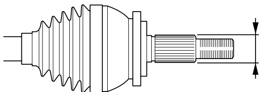
Kuva 1: Oikean pyöränlaakerin tunnistamiseksi on mitattava puoliakselin ulkohalkaisija
