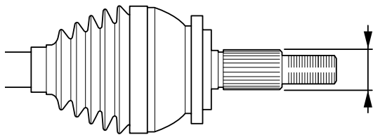
Figura 1: Per l'identificazione del cuscinetto ruota corretto, occorre misurare il diametro esterno del semiasse
