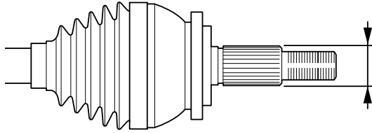
Resim 1: Doğru rulman yatağını tanımlamak için aks mafsalı frezesi şaftının dış çapını ölçün
