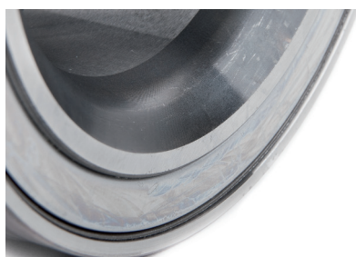
Bild 3: Truck Hub Unit mit Kantenkürzung
