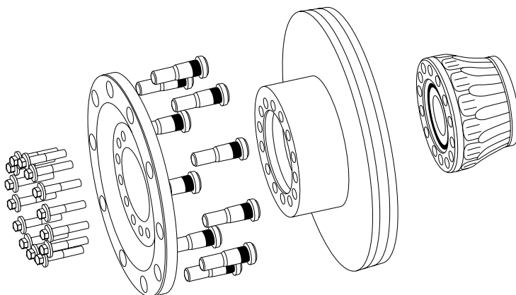
Fig. 1: În cazul punților marcate cu ID-ul S63U, pe lângă modulul rulmentului de roată, trebuie să se înlocuiască și discul de frână, dispozitivul de fixare a roții, prezoanele roților și șuruburile de fixare.
