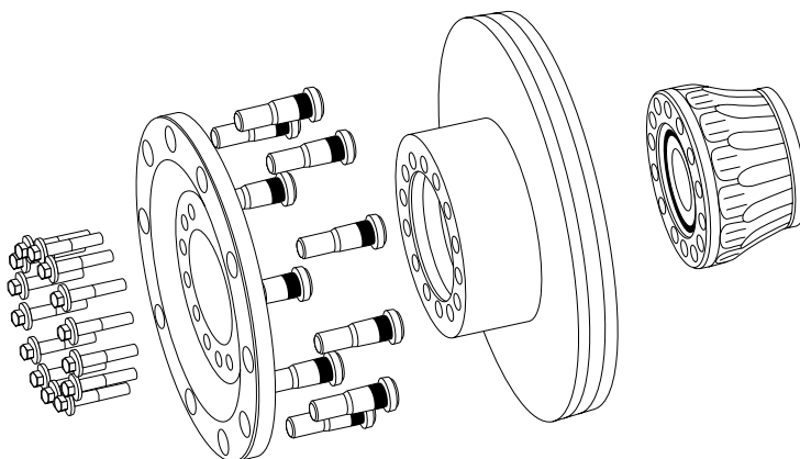
Obrázek 1: U náprav s identifikátorem S63U se musí vedle modulu ložiska kola přídatně vyměnit také brzdový kotouč, uchycení kola, šrouby kola a upevňovací šrouby
