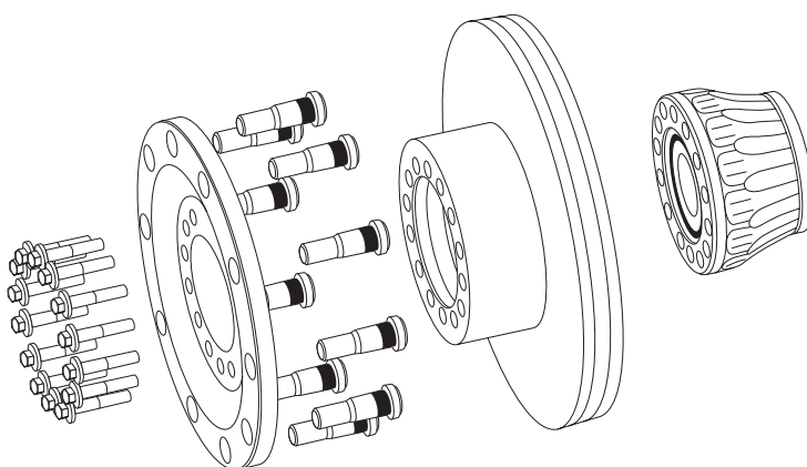
Figura 1: Nel caso di assali S63U, oltre al modulo cuscinetto ruota, occorre sostituire il disco freno, staffa di supporto, il bullone ruota e le viti di fissaggio.
