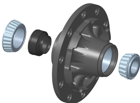
Bild 1: Fettkartusche (schwarz) einer Radnabe für BPW-Achsen
