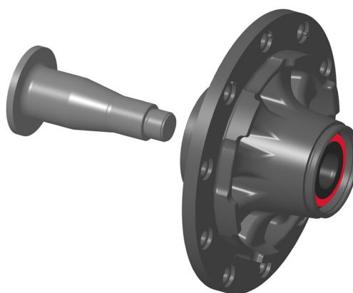
Image 2 : Moyeu de roue avec FAG SmartSET pour essieux BPW
