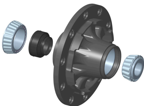
Figura 1: Cartuccia di grasso (nera) di un mozzo ruota per assali BPW
