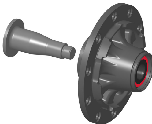
Afbeelding 2: Wielnaaf met FAG SmartSET voor BPW-assen
