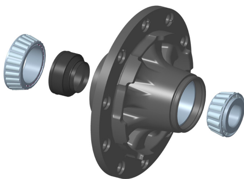
Afbeelding 1: Vetpatroon (zwart) van een wielnaaf voor BPW-assen
