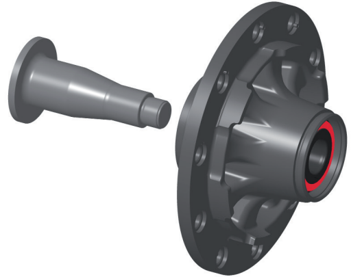
Şekil 2: BPW aksları için FAG SmartSET özellikli tekerlek rulmanı
