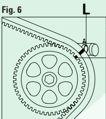
FIGURA 6 Verificar la correcta alineación de las marcas de puesta en fase I con el tornillo L.
