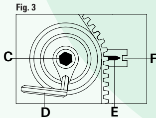
FIGURA 3 Allentare il bullone di bloccaggio C e ruotare in senso orario il tendicinghia, utilizzando la chiave esagonale D, fino ad allineare le tacche di fase E ed F; serrare quindi il bullone di bloccaggio C.
