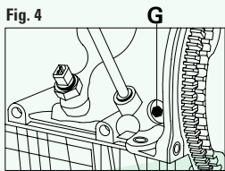
FIGURA 4 Smontare il bullone G ed inserire al suo posto l'attrezzo di bloccaggio H. FIGURA 5 Inserire l'apposito attrezzo di bloccaggio dell'albero motore H e ruotare l'albero motore fino a alla battuta contro il perno.
