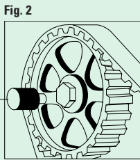
FIGURA 1 Verificar la correcta alineación de las marcas de puesta en fase A. FIGURA 2 Insertar la herramienta especial de inmovilización de árbol de levas B.
