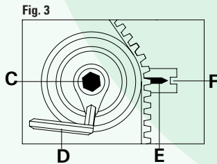
FIGURA 3 Aflojar el tornillo de fijación C. Girar el tensor de correa en sentido de las agujas del reloj, utilizando la llave hexagonal D hasta que las marcas de fase E y F estén en línea. Por último, apretar el tornillo de fijación C.
