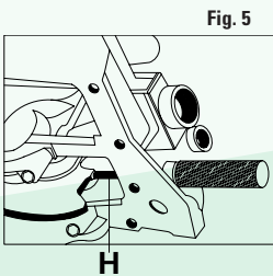
FIGURA 4 Extraer el tornillo G y en su lugar insertar la herramienta de inmovilización H. FIGURA 5 Insertar la herramienta especial para inmovilización de cigüeñal motor H, y girar el cigüeñal hasta que este haga tope contra el perno.
