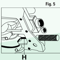
FIGURA 4 Smontare il bullone G ed inserire al suo posto l'attrezzo di bloccaggio H. FIGURA 5 Inserire l'apposito attrezzo di bloccaggio dell'albero motore H e ruotare l'albero motore fino a alla battuta contro il perno.
