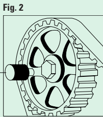
FIGURA 1 Controllare il corretto allineamento delle tacche di fase A. FIGURA 2 Inserire l'apposito attrezzo di bloccaggio dell'albero a camme B.
