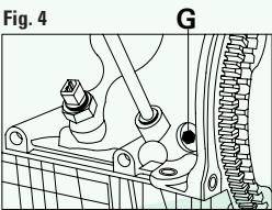
FIGURA 4 Extraer el tornillo G y en su lugar insertar la herramienta de inmovilización H. FIGURA 5 Insertar la herramienta especial para inmovilización de cigüeñal motor H, y girar el cigüeñal hasta que este haga tope contra el perno.
