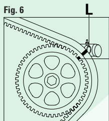
FIGURA 6 Controllare il corretto allineamento delle tacche di fase I con il bullone L.
