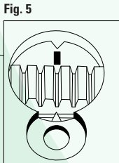
FIGURA 5 Segni di riferimento sul volano: verificare il corretto allineamento delle tacche di fase I.
