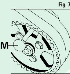
FIGURA 7 Inserire l'apposito attrezzo di bloccaggio della pompa di iniezione M.
