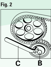
FIGURA 2 Allentare il bullone di bloccaggio B e ruotare in senso orario il tendicinghia utilizzando la chiave C agendo sull'eccentrico di registro.
