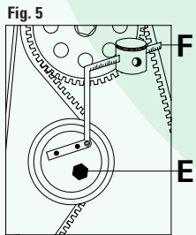
FIGURA 5 Aflojar el tornillo de fijación E, e insertar la herramienta especial de tensado de correa con su relativo peso F (65mm o 70mm). ; Verificar que el brazo de la herramienta se mantenga en posición horizontal; Por último, apretar el tornillo de fijación E.
