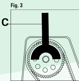
FIGURA 1 Inserire l'apposito attrezzo di comparazione A, sul cilindro N° 1. FIGURA 2 Controllare il corretto allineamento delle tacche di fase B. FIGURA 3 Inserire l'apposito attrezzo C, per mantenere l'ingranaggio in tensione. FIGURA 4 Inserire l'apposito attrezzo di bloccaggio dell'albero a camme D.
