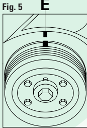
FIGURA 5 Verificar la correcta alineación de las marcas de puesta en fase E.
