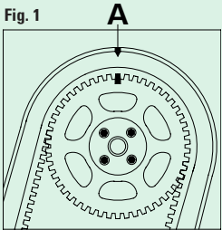
FIGURA 1 Verificar la correcta alineación de las marcas de puesta en fase A.
