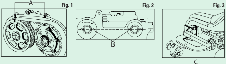
FIGURA 1: Verificar la correcta alineación de los arboles de leva "A". FIGURA 2: Verificar la correcta alineación de los arboles de leva "B". FIGURA 3: Verificar el posicionamiento correcto la herramienta de inmovilización de árbol de levas C.
