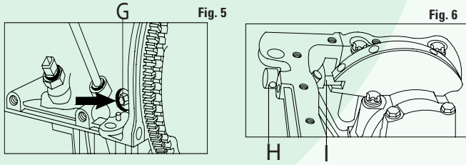
FIGURA 5: Togliere il bullone G dal blocco cilindri. FIGURA 6: Inserire l'apposito attrezzo di bloccaggio dell'albero motore H.
