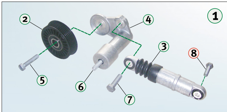
Fig. 1: Reprezentare în detaliu a unității 534 0014 10
