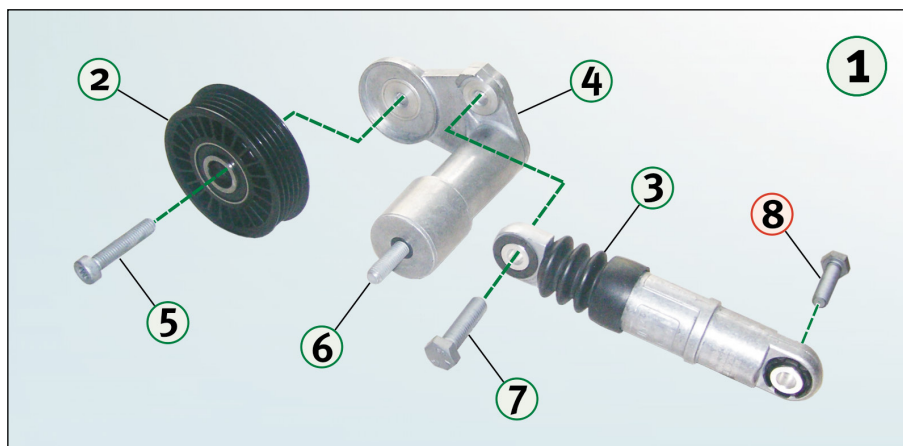
Снимка 1: Подробна илюстрация на 534 0014 10, включваща всичките му компоненти
