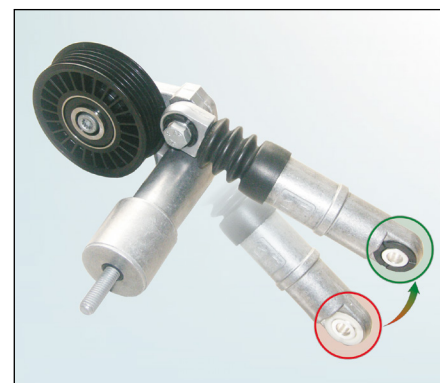
Снимка 2: Версия 534 0014 10, като са показани както черните, така и белите пластмасови втулки на хидравличния демпфер
