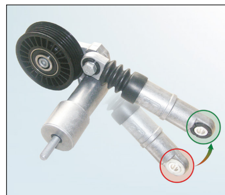
Kuva 2: 534 0014 10 - mallit hydraulivaimentimen kiinnityssilmukkojen valkoisilla ja mustilla muovikoteloilla
