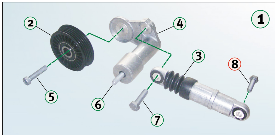
Kuva 1: Yksityiskohtaisesti esitetty 534 0014 10 kaikkine osineen
