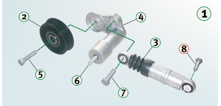
Resim 1: Tüm bileşenleriyle beraber 534 0014 10'un ayrıntılı çizimi
