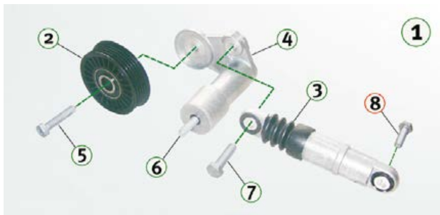
Рис. 1: Детальная иллюстрация узла 534 0014 10, включая все компоненты
