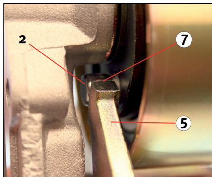
Fig. 3: Poziție corectă (vedere din spate)
