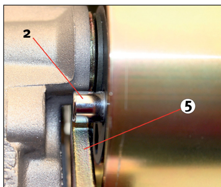
Fig. 5: Poziție incorectă (vedere din spate)
