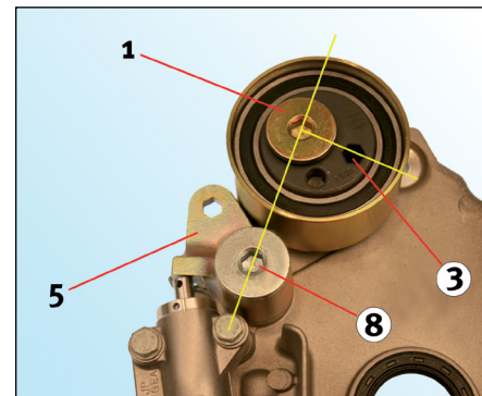
Fig. 4: Poziție corectă (vedere frontală)
