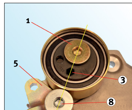
Fig. 6: Poziție incorectă (vedere frontală)
