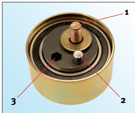
Fig 1: 531 0402 20 (vedere din spate)
