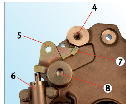
Fig. 2: Capac cilindru
