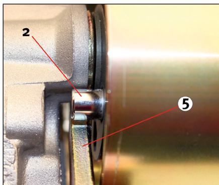
Obrázek 5: Chybná montážní pozice (pohled zezadu)
