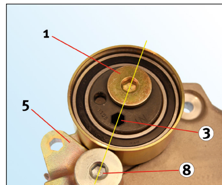
Obrázek 6: Chybná montážní pozice (pohled zepředu)
