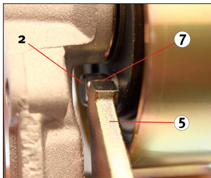
Obrázek 3: Správná montážní pozice (pohled zezadu)
