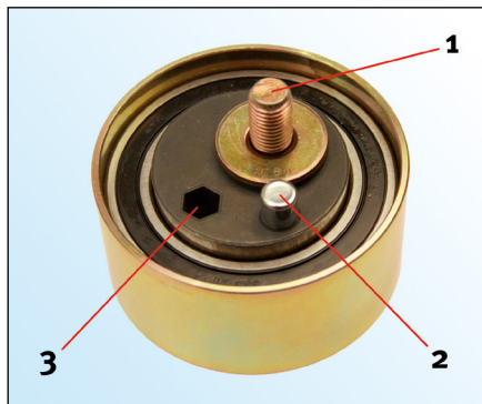
Obrázek 1: 531 0402 20 (pohled zezadu)
