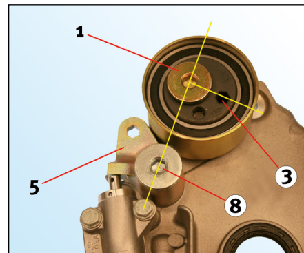
Obrázek 4: Správná montážní pozice (pohled zepředu)
