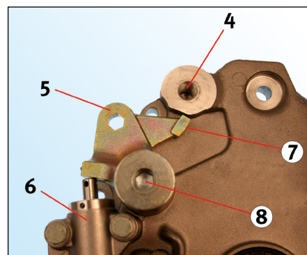
Figur 2: Krumtapakslens lejeskærm
