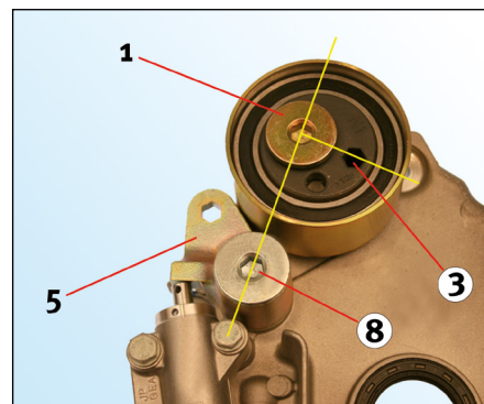
Figur 4: Korrekt monteringsposition (set forfra)
