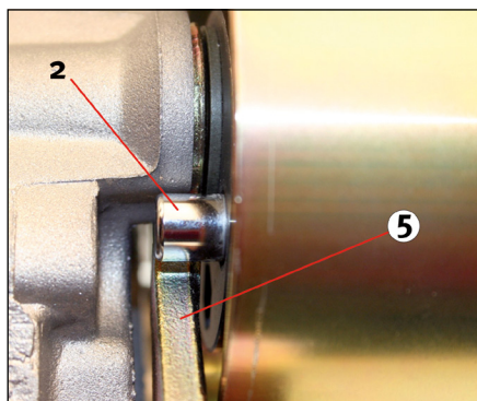
Figur 5: Forkert monteringsposition (set bagfra)
