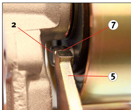
Figur 3: Korrekt monteringsposition (set bagfra)
