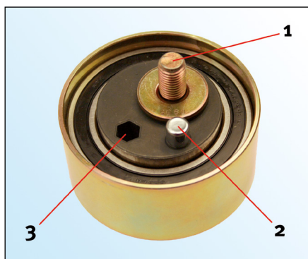
Figur 1: 531 0402 20 (set bagfra)
