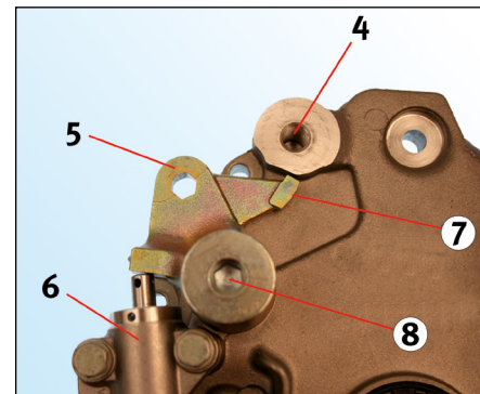
2. ábra: Forgattyútengely csapágyapajzsa
