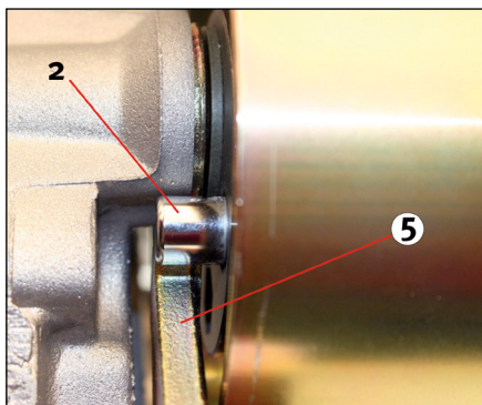
Bild 5: Felaktig monteringsposition (sedd bakifrån)
