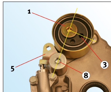
Bild 4: Korrekt monteringsposition (sedd framifrån).
