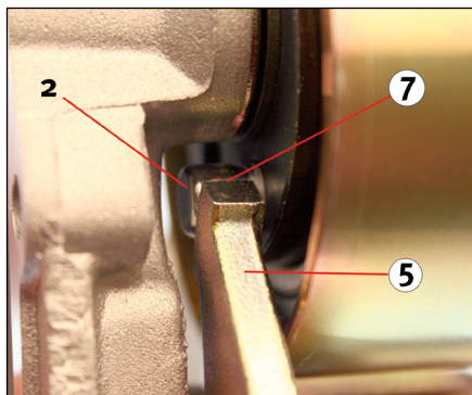
Bild 3: Korrekt monteringsposition (sedd bakifrån).
