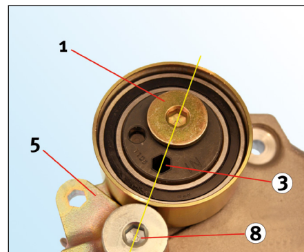
Bild 6: Felaktig monteringsposition (sedd framifrån)
