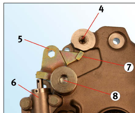
Bild 2: Lagersköld till vevaxel
