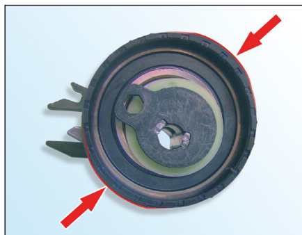
1. ábra: 531 0564 30 (Előlnézet)
