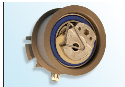
Bild 2: 531 0565 30 (nytt utförande)
