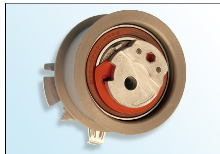
Εικόνα 2: 531 0628 30 (νέα παραλλαγή)
