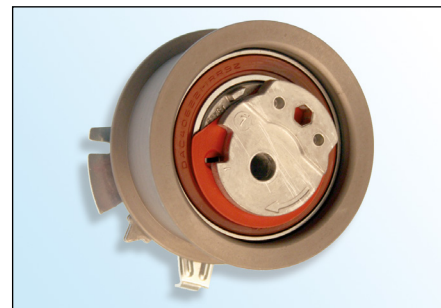
2. ábra: 531 0628 30 (új kivitel)
