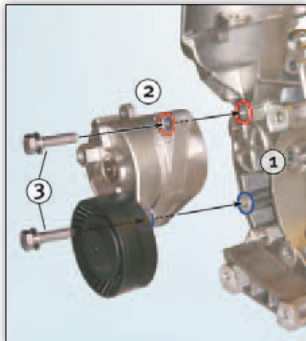
Снимка 4: Монтажно положение на механичното обтягащо рамо
