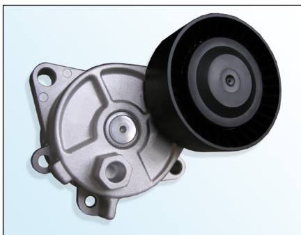
Kuva 1: 533 0015 10 mekaaninen kiristinvarsi
