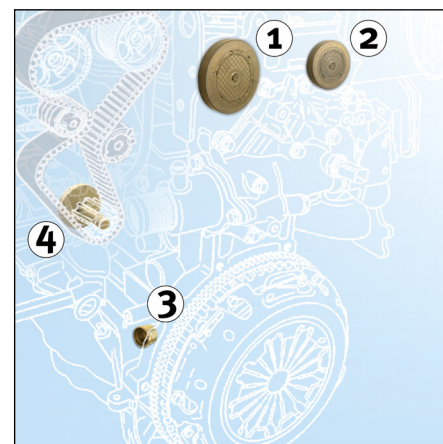
Figura 2: Poziție montare
