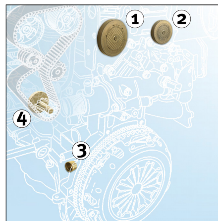
Снимка 2: Монтажна позиция
