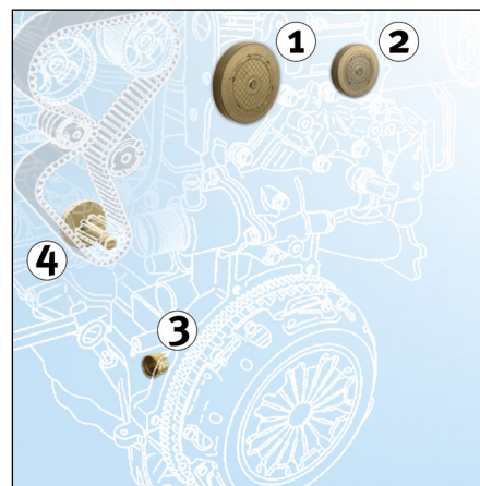
Fig. 2: Monteringsposition
