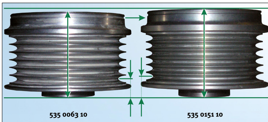
Imagine 3: Deosebirea roților libere pentru alternator INA 535 0063 10 (VALEO) și 535 0151 10 (DENSO)
