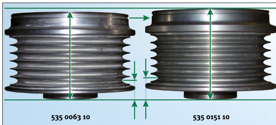
Figur 3: Adskillelse mellem friløbshjul til generator INA 535 0063 10 (VALEO) og 535 0151 10 (DENSO)
