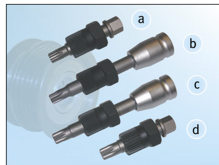
Figur 2: Oversigt af specielværktøj
