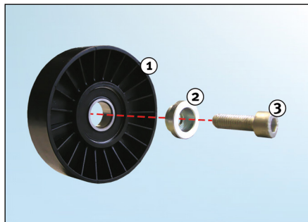
Снимка 1: 532 0138 10 – предишна конструкция
