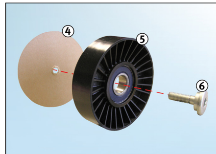
Снимка 2: 532 0138 10 – нова конструкция
