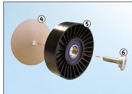
Obr. 2: 532 0138 10 - nové provedení
