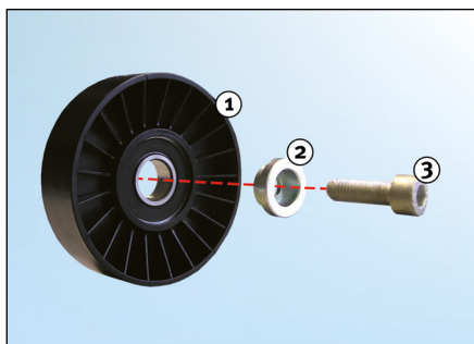
Fig. 1: 532 0138 10 - gammel udførelse
